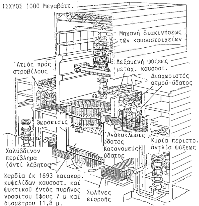
ΓΕΝΙΚΗ ΑΠΟΨΙΣ ΤΟΥ ΑΝΤΙΔΡΑΣΤΗΡΟΣ ΓΡΑΦΙΤΟΥ ΕΙΣ ΤΣΕΡΝΟΜΠΙΛ ΙΣΧΥΟΣ 1000 Μεγαβάττ.
