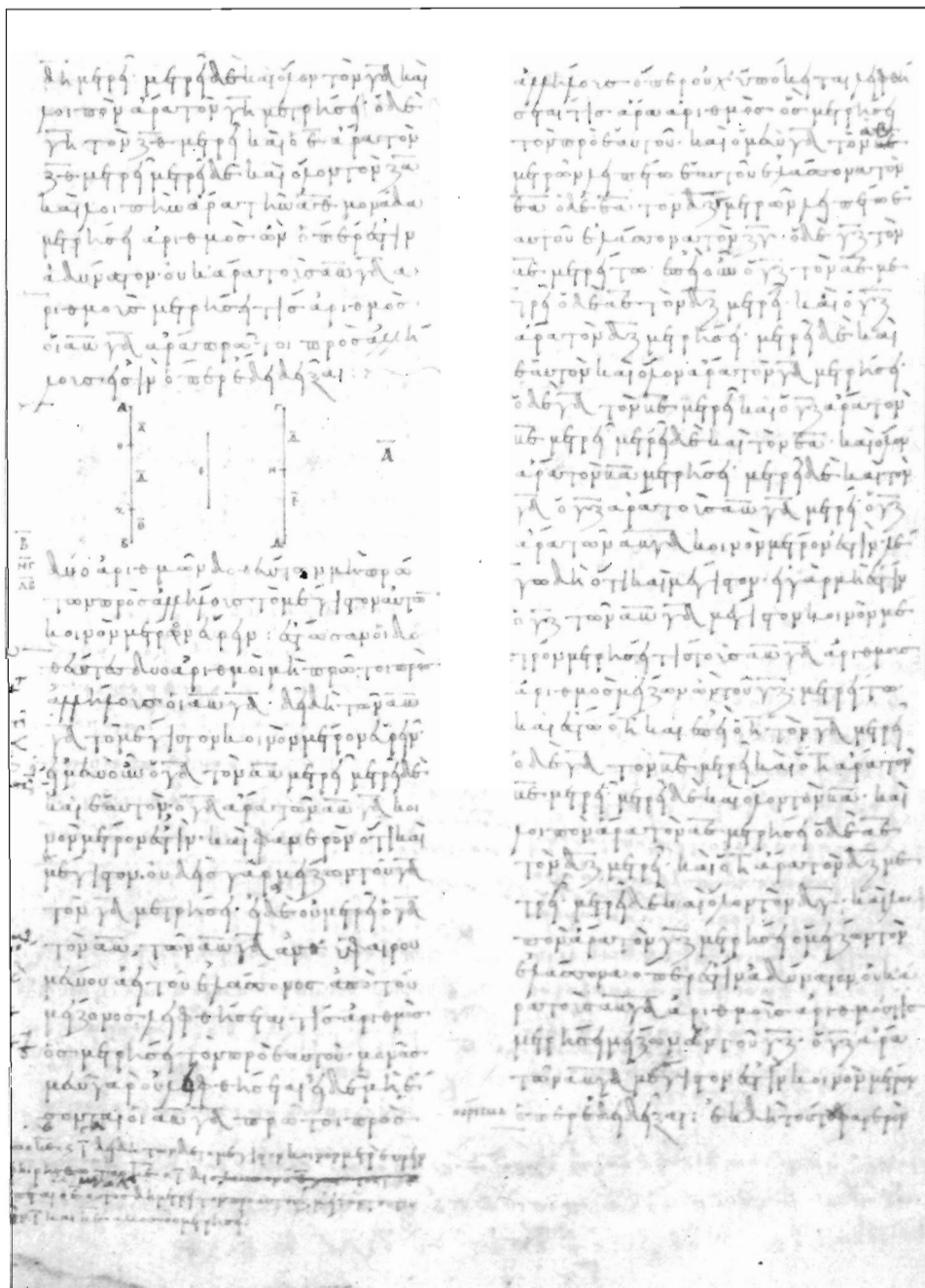
Ὁ ἀρχαιότερος ἀλγόριθμος: Σελίδα χειρογράφου τοῦ 10ου αἰῶνος τῶν «Στοιχείων» τοῦ Εὐκλείδου (3ος π.Χ. αἰών). Χρησιμοποιεῖται ἀκόμη σήμερα ἀπὸ τοὺς ἐπιστήμονες τῆς πληροφορικῆς στὸ πρόγραμμα “BASIC”!
