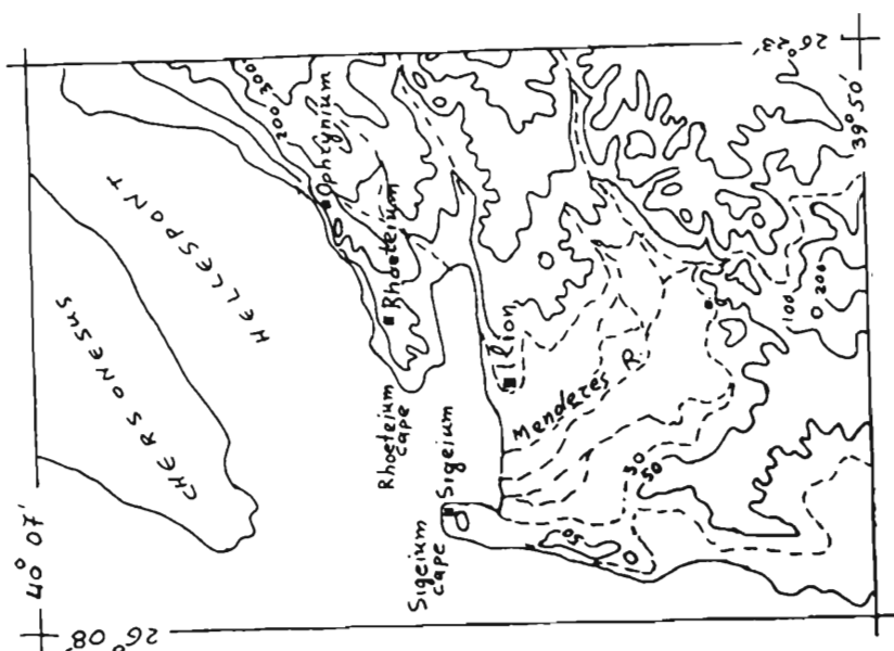
Σχήμα 3: Κλίμαξ 1: 250.000. Χάρτης της Τρωάδος, όπως ήταν κατά την έποχή του Ήροdotου (450 π.Χ.)
