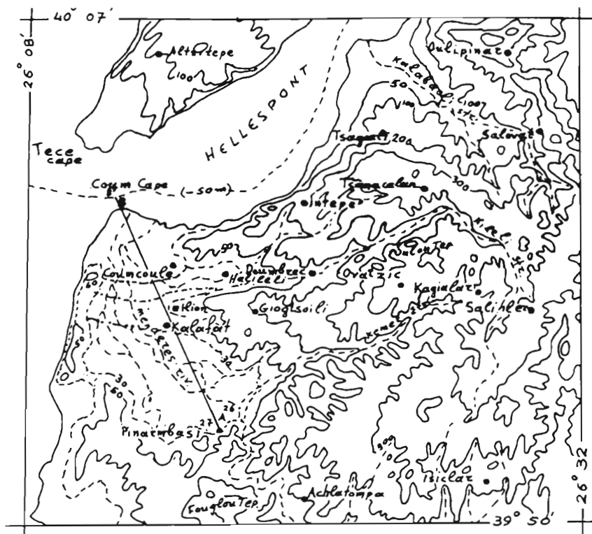
Σχήμα 1: Κλίμαξ 1:250.000. Ο σημερινός χάρτης της Τρωάδος.
