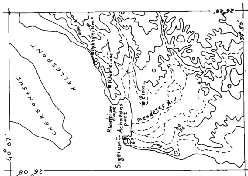
Σχήμα 2: Κλίμαξ 1: 250.000. Χάρτης της Τρωάδος, όπως ήταν κατά την εποχή του Στράβωνος (105 αι. μ.Χ.)
