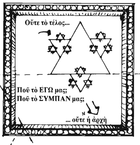
Σχ. 2. Ἀπλὸ fractal (κλασματομορφή) (ἀπείρως μικρὸ / ἀπείρως μεγάλο).
