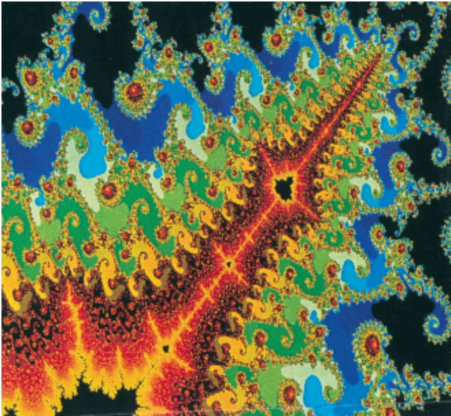
Ἕνα ἀπὸ τὰ φράκταλς: Τὸ σύνολο Mandelbrot.
