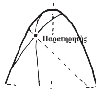
Σχ. 1. Χῶρος Riemann.
