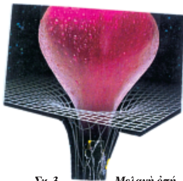
Σχ. 3. Μελανὴ ὀπή.
