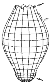
Σχ.1. Μορφή Big Bang.
