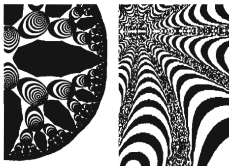
Σχ.3. Κλασματομορφές ( fractals ).
