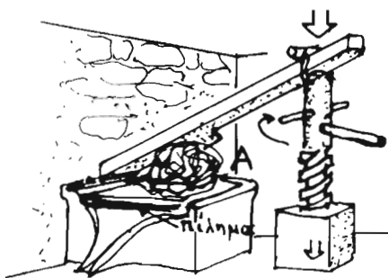
Σχ.2. Πιεστήριος έλιξ γναφείου κατά Gille.
