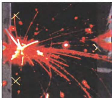
Φωτ. 3. Τροχιές ύποατομικών σωματιδίων.
