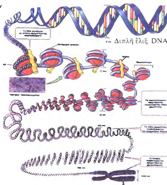
Σχ. 5. Το DNA στο χρωμόσωμα - άνελισσόμενη έλιξ.
