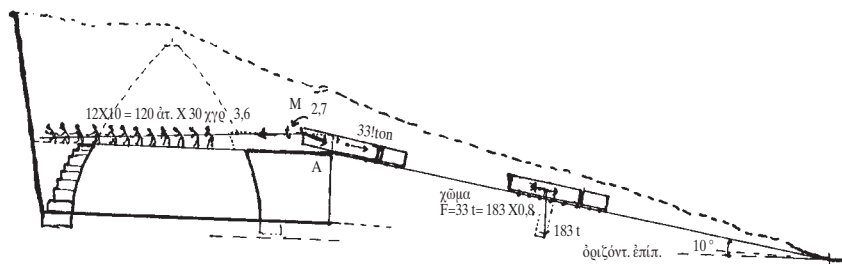
Σχ. 6. Ἀδύνατη ἢ ἀνύψωση τοῦ ὑπέρθυρου μέ κεκλιμένο ἐπίπεδο.
