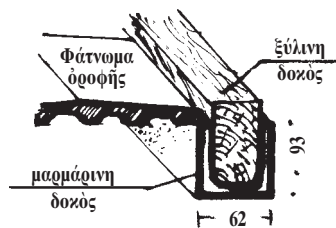
Σχῆμα 7. Τεχνικὴ τῆς θεμελίωσης.
