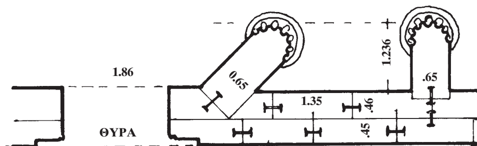
Σχήμα 3. Αντηρίδες και τοίχος του σηκού.
