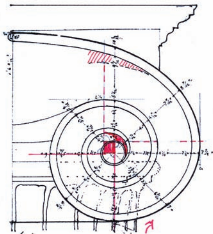
Σχήμα 8. Ἴωνικό κιονόκρανο.
