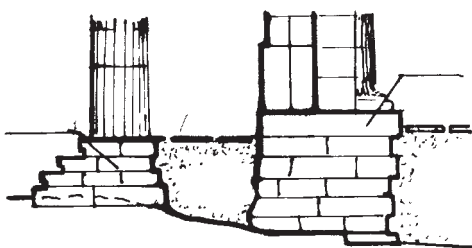
Σχῆμα 5. Τομὴ θεμελίωσης.
