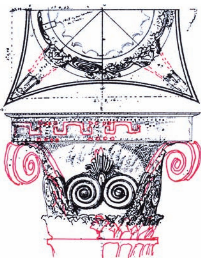
Σχήμα 9. Κορινθιακό κιονόκρανο.
