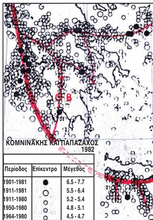
Σχήμα 4. Σεισμικός χάρτης τῆς Νότιας (ἡπειρωτικῆς) Ἑλλάδος.
