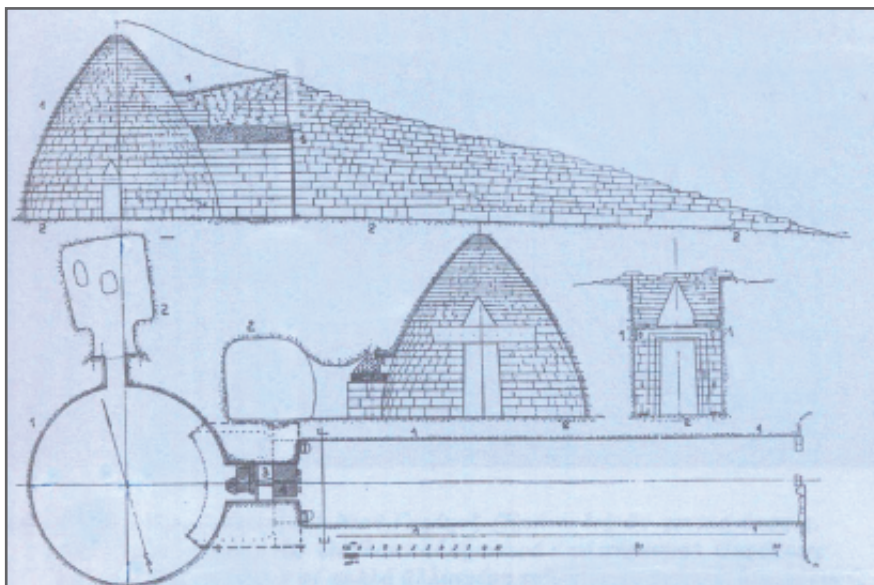
Εἰκόνα 2. Κάτοψη τοῦ «Θησαυροῦ τοῦ Ἀτρέως».
