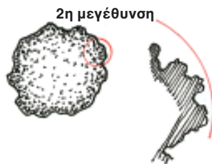
Σχ. 2. Μεγέθυνση ἐνὸς «σημεῖου».
