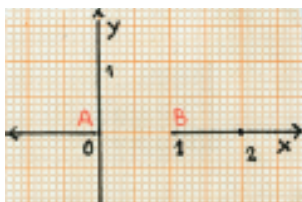
Σχ. 3. Η «μονάδα» AB \approx 1 .
