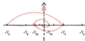
Σχ. 1. Παράσταση \text{ὄρ}(-1)^v \cdot \frac{1}{2^v} = 0 .
