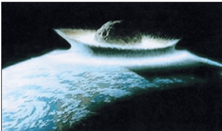
Εἰκόνα Α: Ἀναπαράστασις σὲ Η/Υ πτώσεως μετεωρίτου ἐπὶ τῆς Γῆς. Ἡ πῶσις ἐνὸς μετεωρίτου μὲ μέγεθος ὡς τοῦ εἰκονιζομένου, εἶναι ἀρκετὴ νὰ καταστρέψῃ ὄχι μόνο τὸν πολιτισμὸ ἀλλὰ καὶ ὅλη τὴ ζωὴ ἐπὶ τῆς γῆς.
