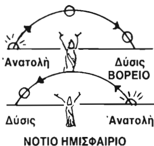
Σχ. 4. Πῶς βλέπουν τὸν ἥλιο οἱ δύο παρατηρητές.
