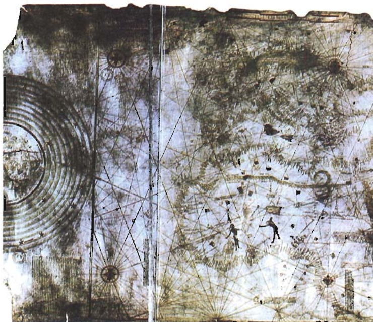
Άνω: Χάρτης Α. Ο χάρτης του Χρ. Κολόμβου. Κάτω: Χάρτης Β. Αεροφωτογραφία από ύψος 35,908 χλμ. (με μαύρη γραμμή) και ο Χάρτης Α του Κολόμβου (με κόκκινη γραμμή). Το μπλε ορθογώνιο έπικολλημένη αερογραφία της περιοχής Μεσογείου.
