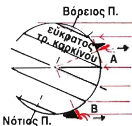
Σχ. 2. Γῆ τὴν 22 Ἰουνίου.
