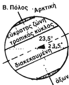
Σχ. 5. Κύκλοι καὶ Ζώνες.
