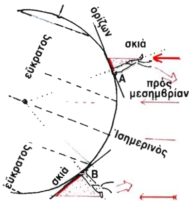
Σχ. 3α. Οἱ σκιὲς Βορ. Εὐκράτης ζωῆς καὶ Νοτίου.
