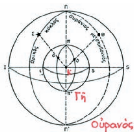
Σχ. 1. Ἀξονας καὶ πόλοι τοῦ κόσμου καὶ τῆς Γῆς.
