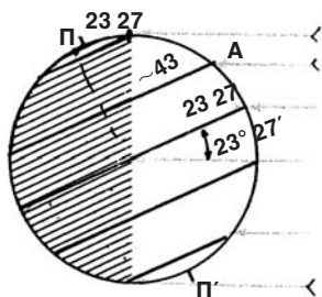
Σχ. 3. Οί ζώνες.
