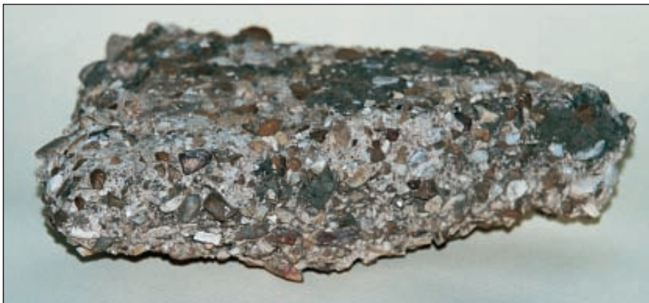
Κομμάτι «μπετόν» από την ύδατοδεξαμενή της αρχαίας Παλαίρου. Ἔχει πάχος τριῶν περιέπου ἐκατοστών. Τὰ ἀδρανῆ υἷλικά του (χαλίγια) ἐμφανίζουn τρία χρώματα (καφέ, μπέζ καὶ ἄσπρο), ἐνῶ τὸ χρώμα τοῦ συνδετικοῦ υἷλικου εἶναι ἀκριβῶς ἴδιο μὲ τὸ τοῦ σημερινοῦ τσιμέντου.
