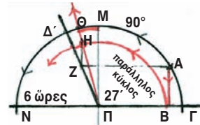
Σχ. 11. Κάτοψη Γῆς ΑΓ= Πλάτος σὲ μοῖρες ΓΜΘ = ΘΜ + 12ω = ὥρες μέγιστης ἡμέρας.
