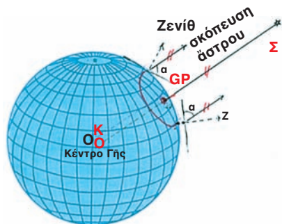
Σχ. 2. Γεωγραφικὴ θέση GP. Ἡ γήινη προβολὴ οὐρανοῦ σώματος.
