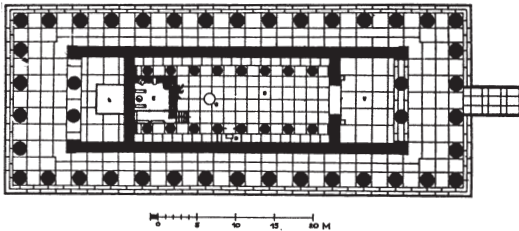
Σχ. 14. Έκτος ναός τοῦ Ἀπόλλωνα. 366-320 π.Χ. Κάτοψη.
