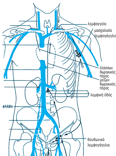
Σχ. 3. Λεμφοφλεβικὴ κυκλοφορία.
