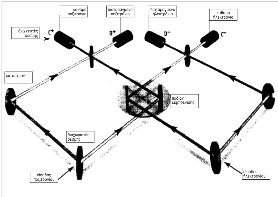
Εικόνα 1. Το «Παράδοξο του Χάρντυ». Το ηλεκτρόνιο και το ποζιτρόνιο, εισερχόμενα στο «πεδίο εκμηδένισης», θα έπρεπε να εξουδετερωθούν. Όμως παραδόξως συνεχίζουν να εμφανίζονται στους ανιχνευτές D. (Σχέδιο του περιοδικού «New Scientist», Μάιος 2003).
