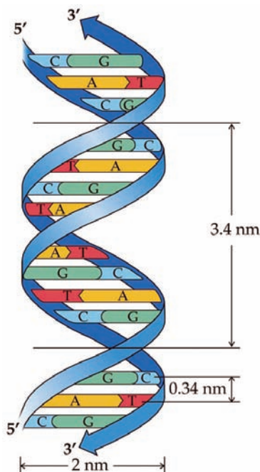
Σχ. 1. Διπλή σπείρα DNA.
