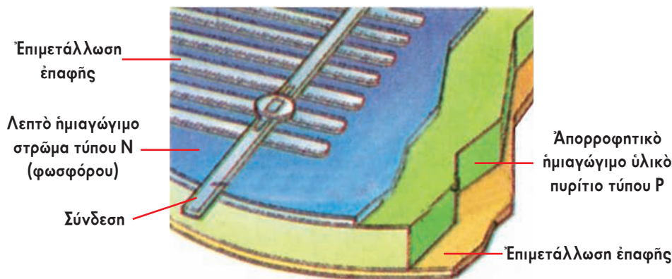
Κατασκευαστική λεπτομέρεια φωτοστήλης πυριτίου.
