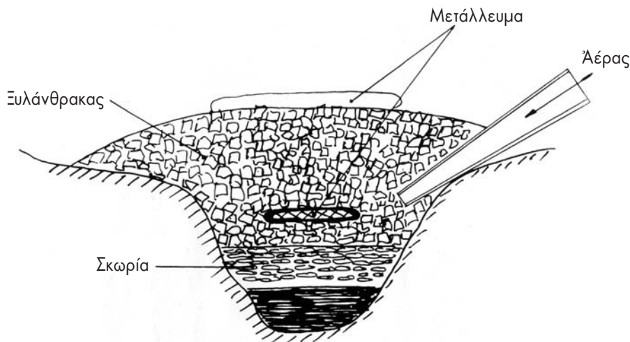
Πρωτόγονος λαγκοειδής κλίβανος παραγωγής μετάλλων. Στόν πυθμένα συλλεγόταν τὸ βαρὺ μέταλλο.
