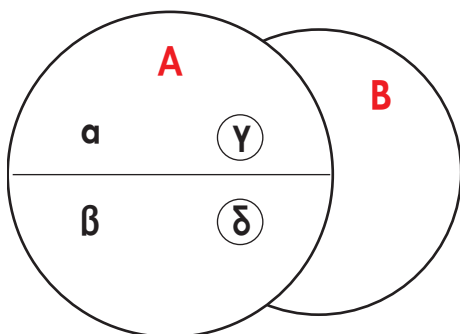
Σχ. 1. Σύνολα ἀριθμῶν.
