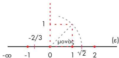
Σχ. 2. Ρητοὶ καὶ ἄρρητοι ἀριθμοὶ ἐπ' εὐθείας.
