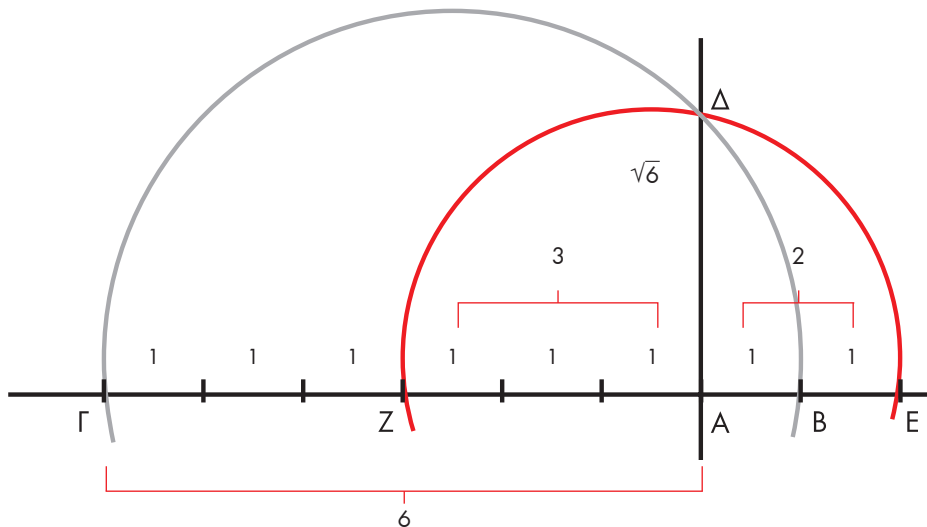
Σχ. 8. Κατασκευή του AA = \sqrt{6} με δύο τρόπους.
