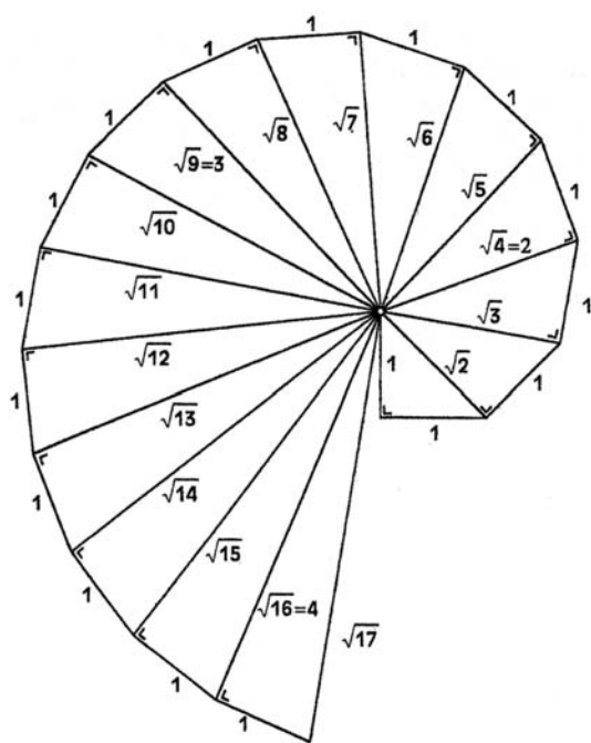
Σχ. 6. Μέθοδος τοῦ Θεοδώρου (;) ἀπὸ τὸν H. Kracke (1968).
