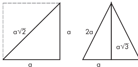
Σχ. 3. Τετρ. ρίζες τοῦ 2 καὶ 3.
