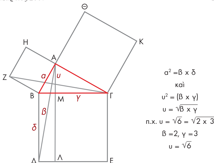
Σχ. 7. Θεώρημα Πυθαγόρα. Επίλυση με θεώρημα Εὐκλείδη.
