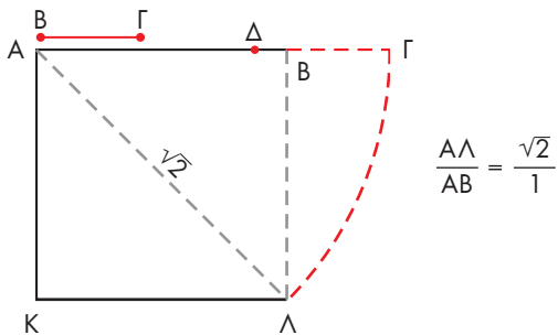
Σχ. 5. Εύρεση της \sqrt{2} δι' ἀνθυφαιρέσεως.
