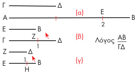
Σχ. 4. Μέθοδος άνθυφαιρέσεως.
