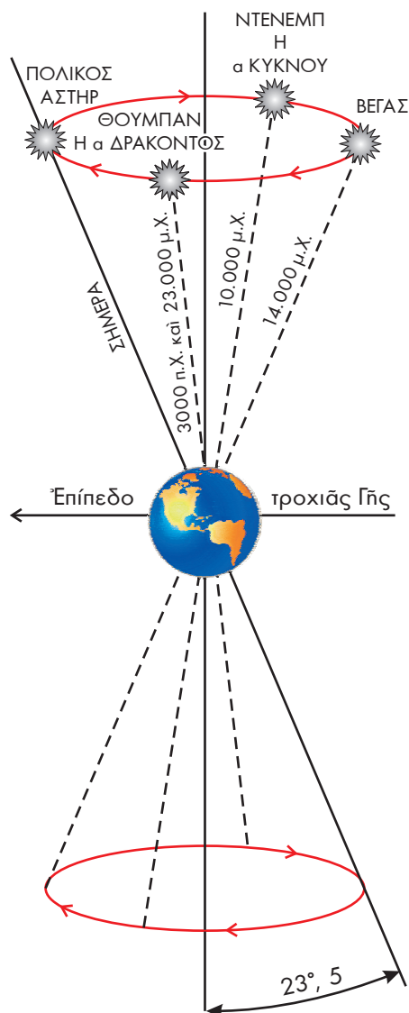
Σχ. 2. Οἱ ἐκάστοτε πολικοὶ ἀστέρες λόγῳ τῆς μεταπτώσεως τῶν ἰσημεριῶν.
