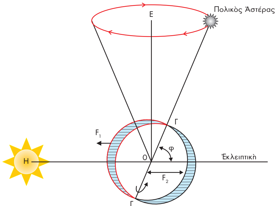
Σχ. 4. Η συνισταμένη τῶν δυνάμεων F_1 καὶ F_2 προκαλεῖ μετάπτωση τοῦ ἄξονα τῆς Γῆς.
