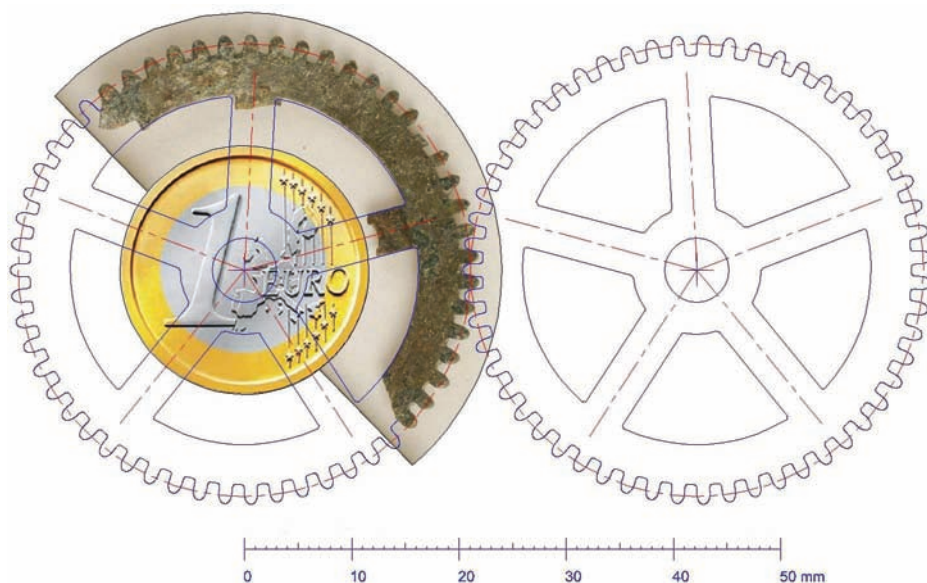
Τὸ Γρανάζι τῆς Σαρδηνίας μὲ ἐμφανῆ τὴν καμπυλότητα ὁδόντωσης. Ἡ ἐντυπωσιακὴ ὁμοιότητά του σὲ σχῆμα καὶ διαστάσεις μὲ τὰ γρανάζια τῆς σύγχρονης Τεχνολογίας ἐγίνε ἀντιληπτὴ μετὰ τὴν ἀποκατάσταση καὶ τὴν ἀκριβῆ γραφικὴ ἀναπαράστασή του στὸν ὑπολογιστὴ. (Φωτογραφία, σχέδιο: Τζιοβάννι Παστόρε.)
